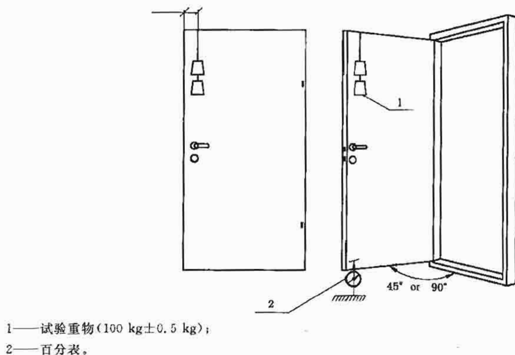
图 4 悬端吊重试验
