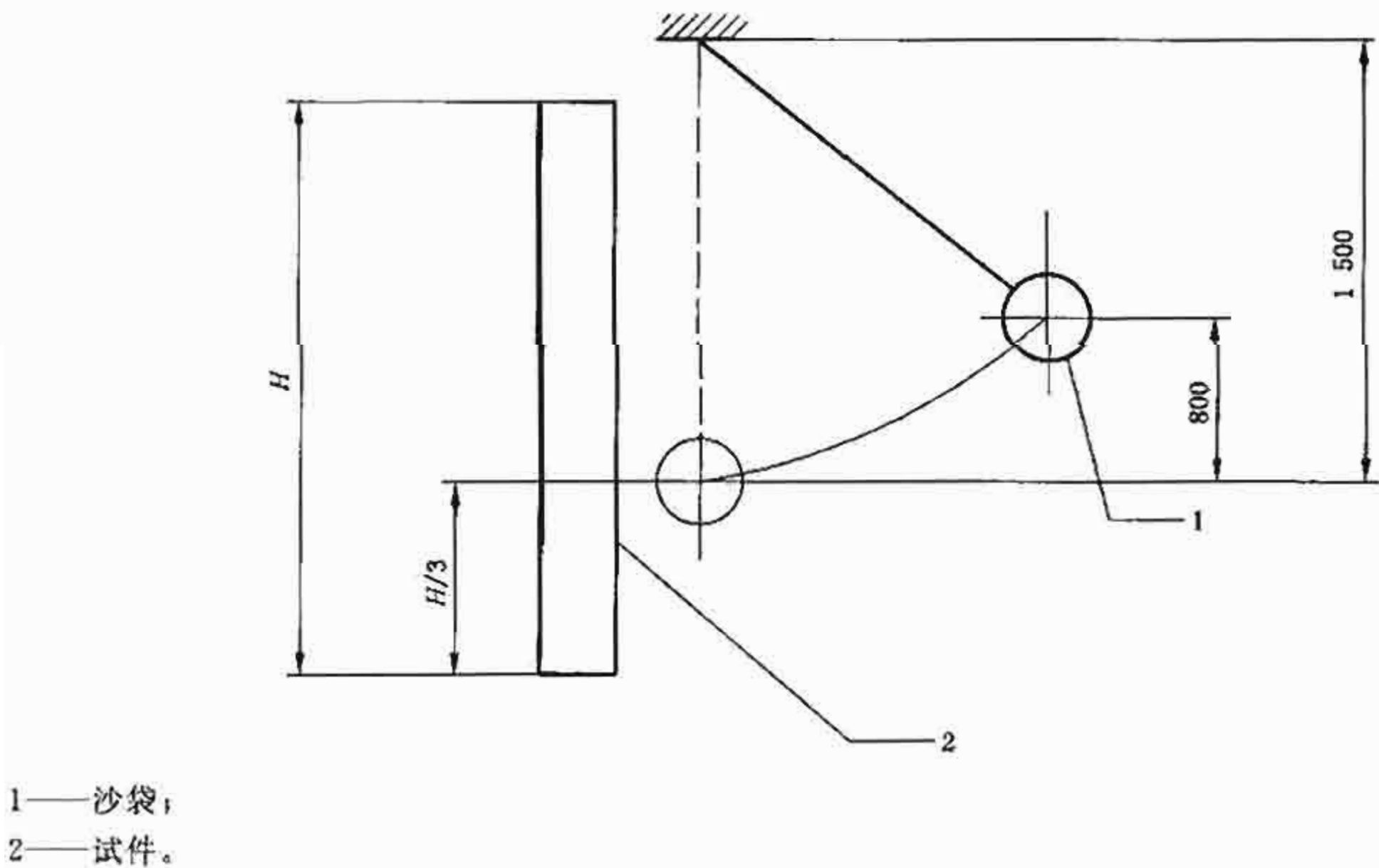
图 3 软冲击试验
