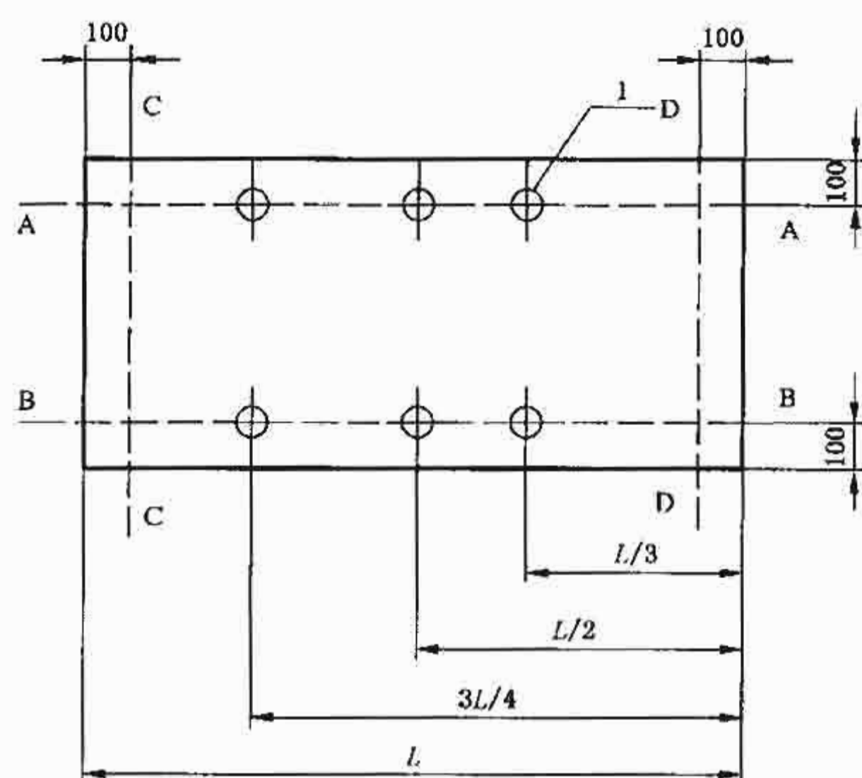
图 1 尺寸公差测量
