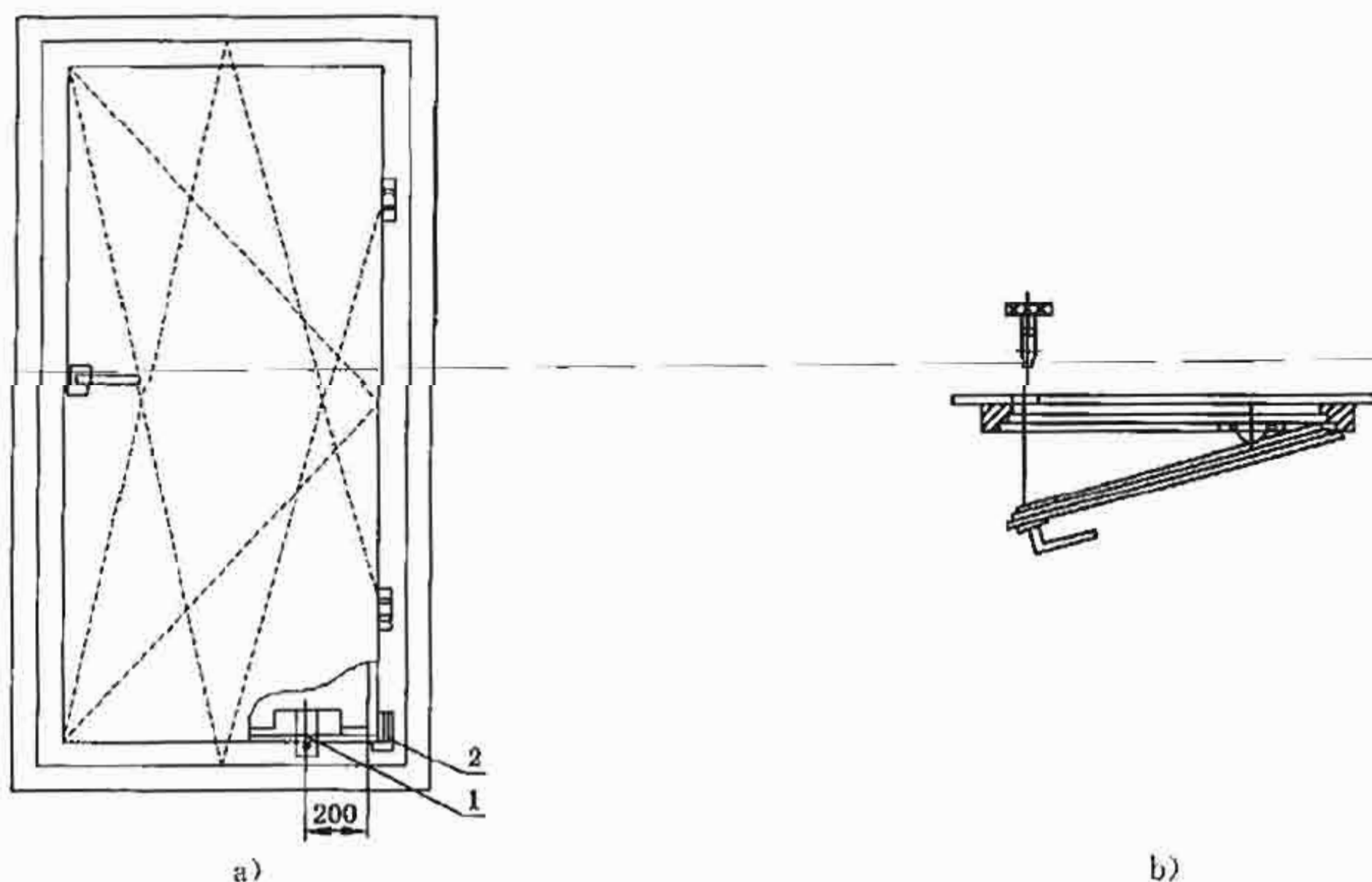
图 5 撞击障碍物试验
