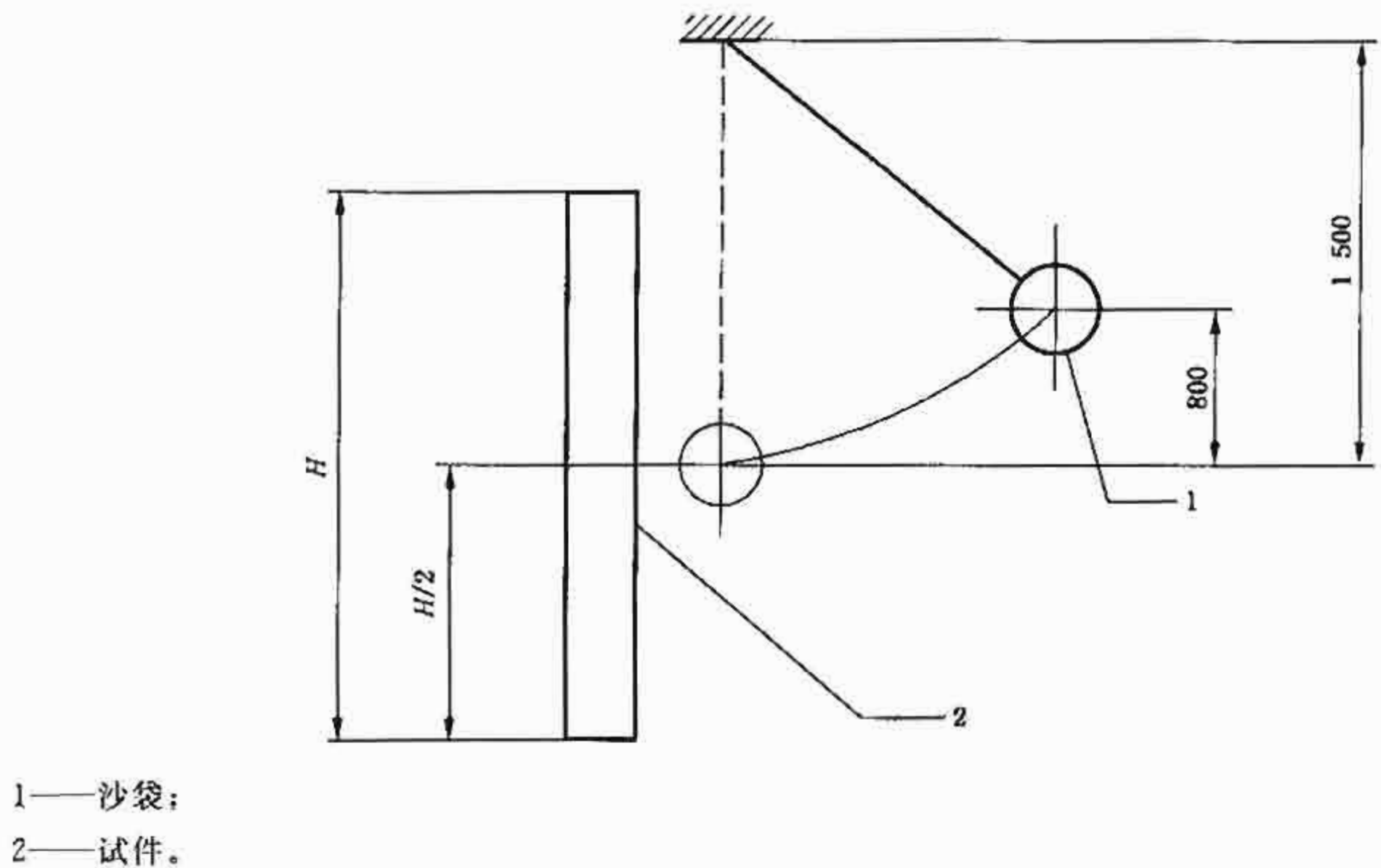
图 2 防闯入试验
